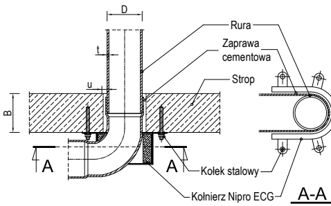
Rys. Przejście kabli w rurze PVC przez strop zabezpieczone kolierzem Nipro ECG.
